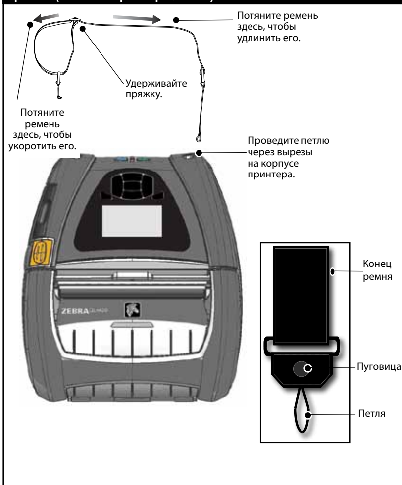
Рисунок 32. Использование дополнительного наплечного ремня (показан принтер QLn420)
