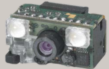
SE4500 2D Imager Module
